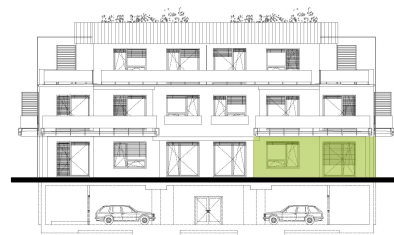
Pohled jihozápadní
