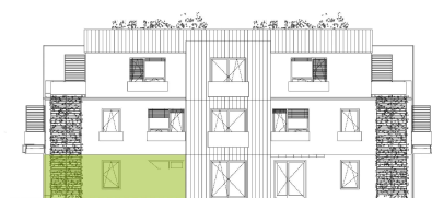
Pohled severozápadní
